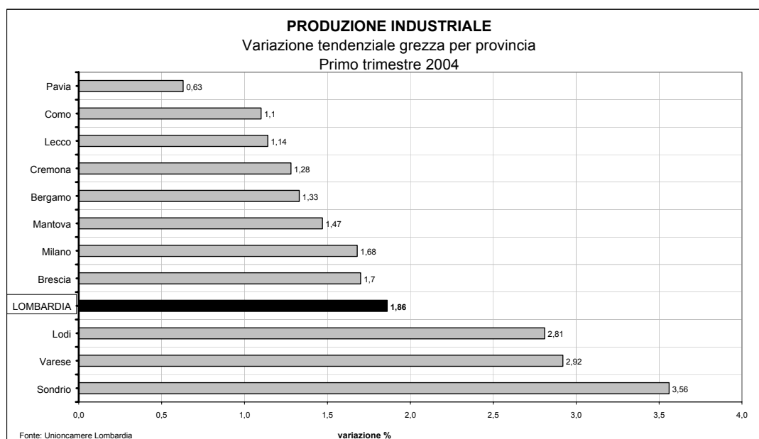
Grafico 2: Produzione industriale: variazione tendenziale grezza per provincia
