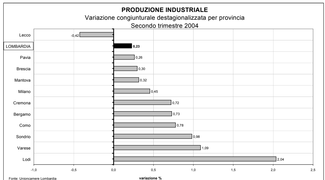
Grafico 1: Produzione industriale destagionalizzata. Variazione congiunturale per provincia
